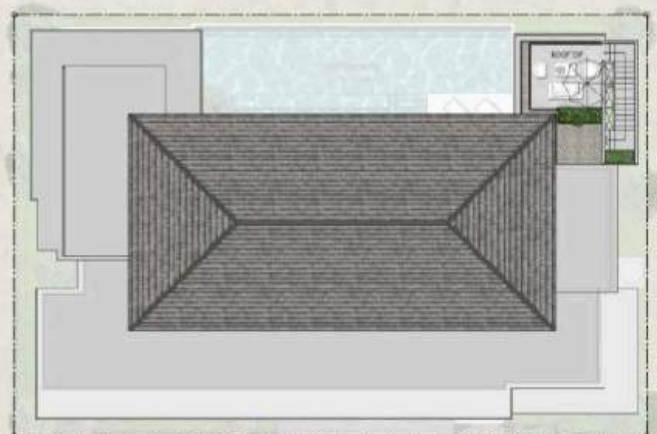
План крыши
