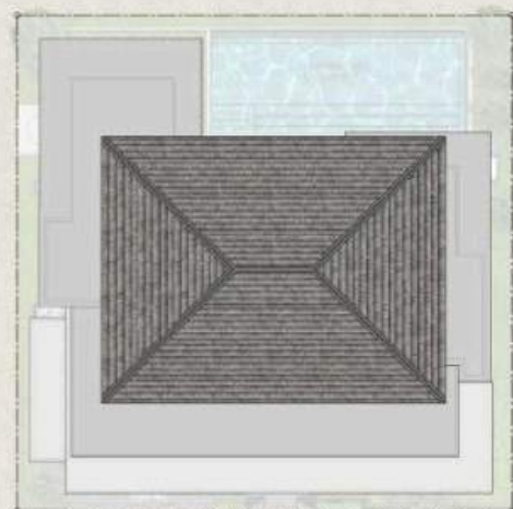
План крыши
